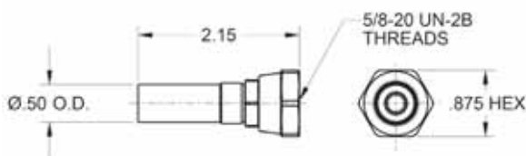
Aeroquip Adapter Assembly
